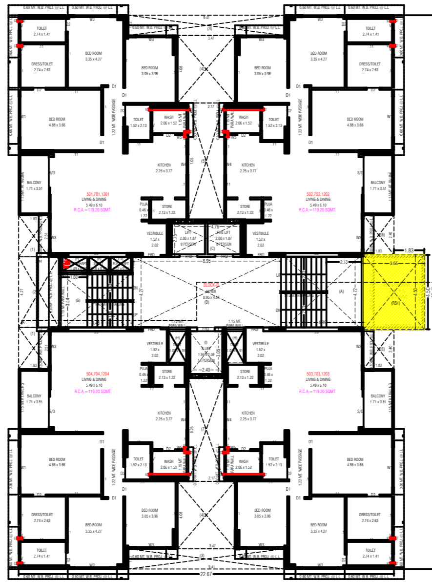
5TH.FL.,7TH.FL.,12TH.FLOOR PLAN
