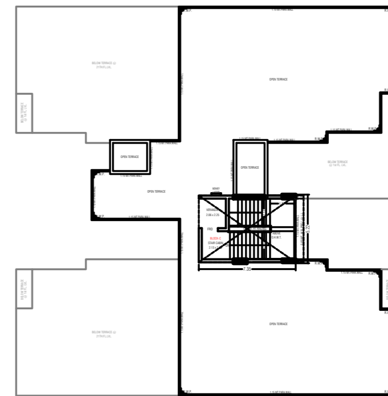
OPEN TERRACE PLAN (STAIR CABIN, O.H.W.T.)
